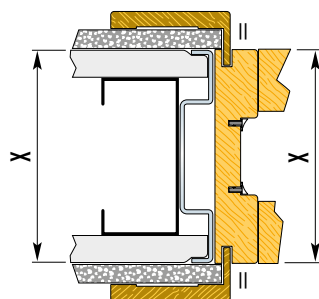
Instalação com alizar regulável
